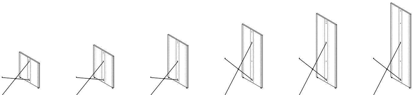
Doppelseitige mittlere Sektion - H720/920/1220/1520/1820/2120 mm
