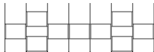
7 doppelseitige Sektionen = 9 Rahmenraverse
