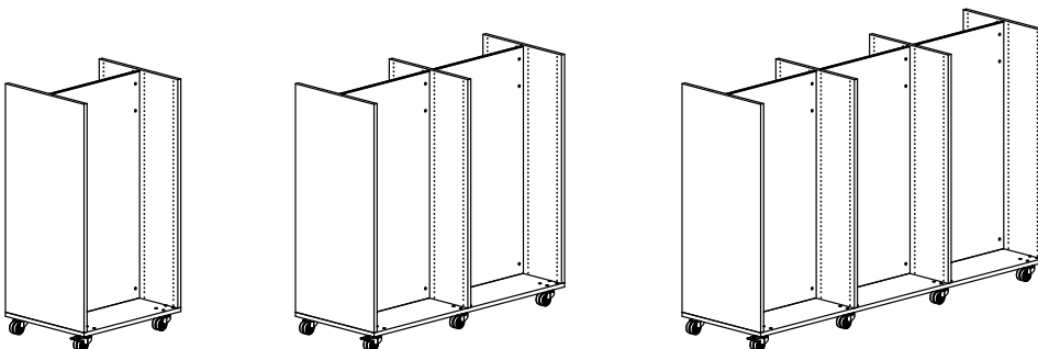
Doppelseitiges Regal - H1520 mm - 1/2/3 Sektionen
